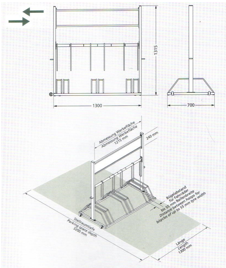
Sicherer und platzsparender Beidseitiger Radeinstand.
