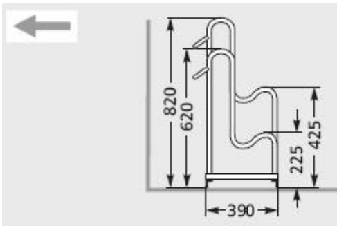
Modellreihe 4000 BR
