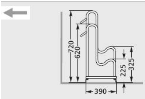
Modellreihe 4000
